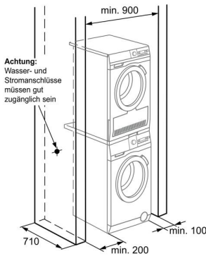
Belüftungsbeispiel für Wasch-Trockensäule, Nischeneinbau
